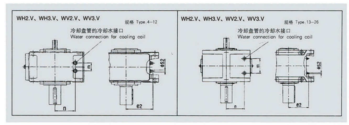
齿轮箱冷却盘管尺寸图 立式安装
