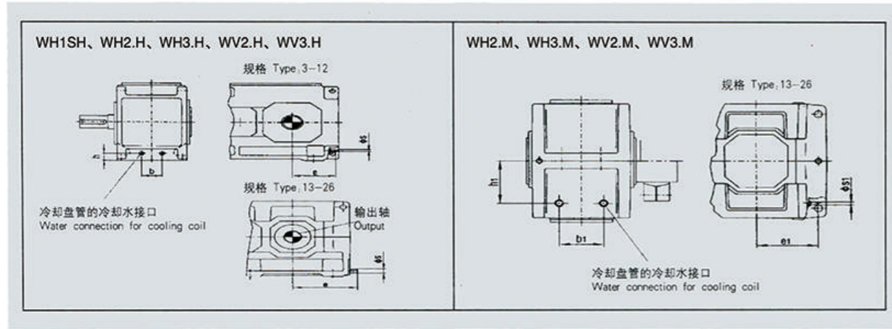
齿轮箱冷却盘管尺寸图 卧式安装
